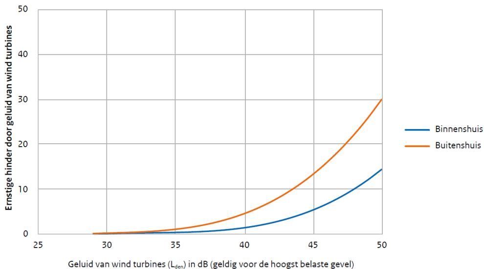
Figuur 4. Relatie tussen geluid van windturbines L_{den} (op de gevel, buitenshuis) en het percentage ernstig gehinderden binnenshuis en buitenshuis door windturbines (Janssen et al., 2008, overgenomen uit Welkers et al., 2020).
